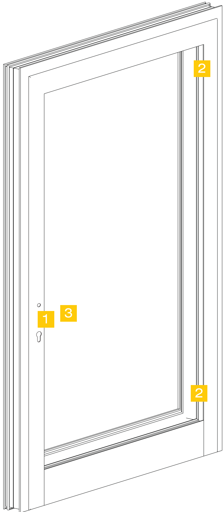
Hinge 2 1121 - 1122.200
