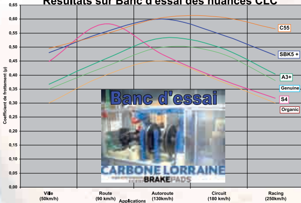
Résultats sur Banc d'essai des nuances CLC
