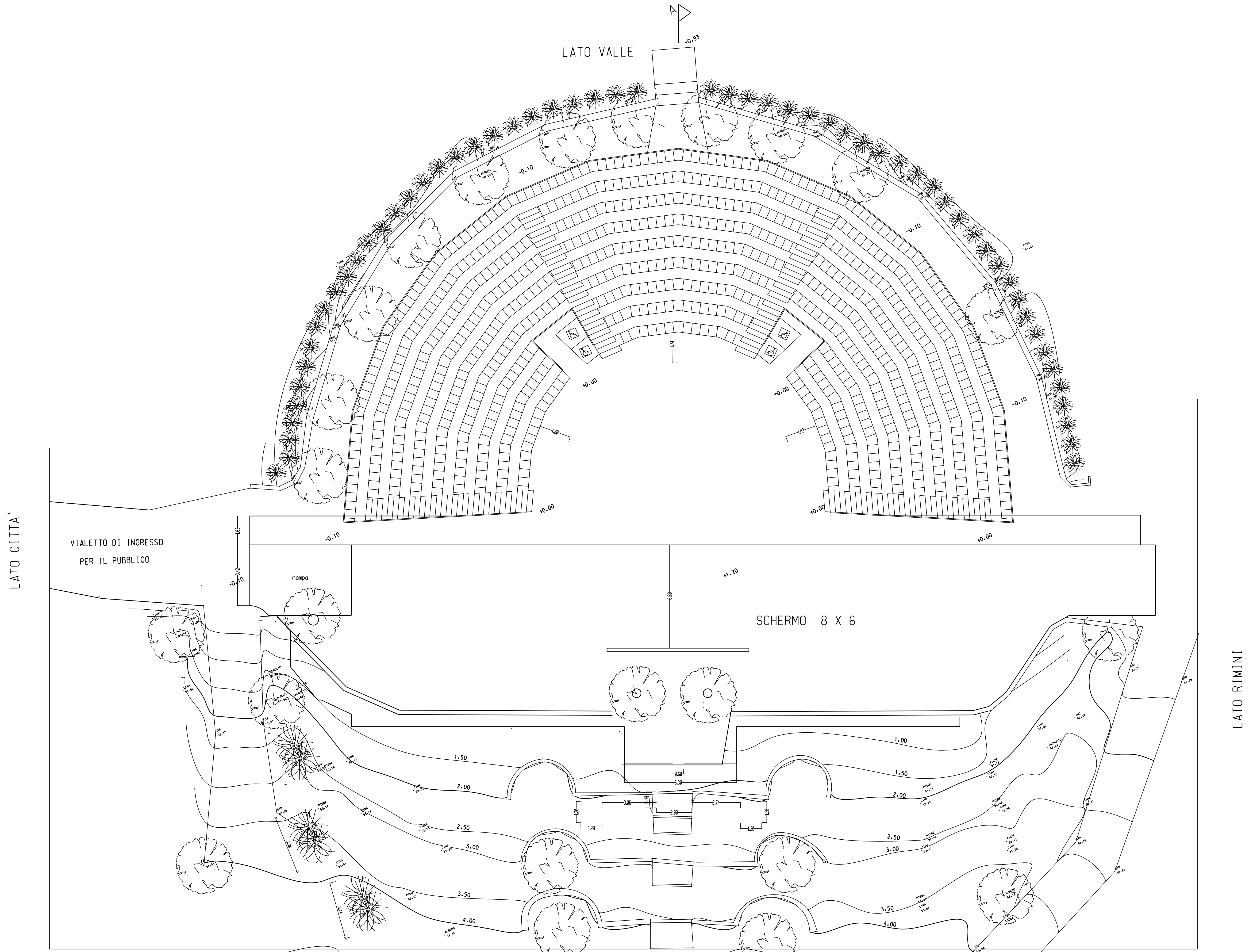
PIANTA
