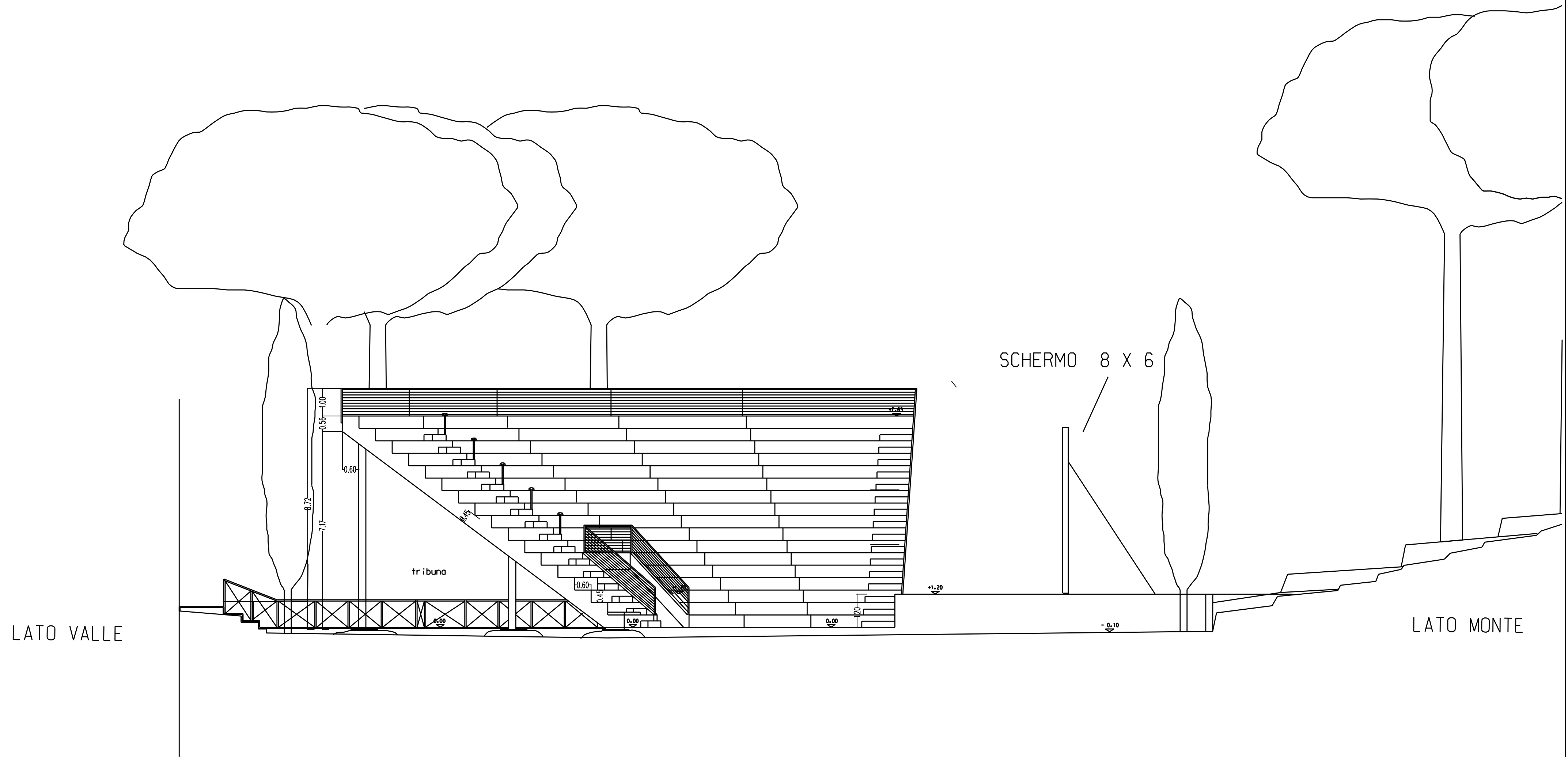
SEZIONE A-A
