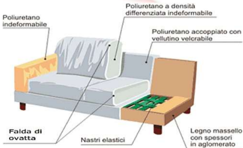
Fig.1 - Struttura di un divano
